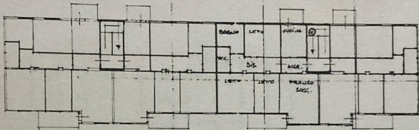
PIANTA PIANO 1 o h. 2.70
